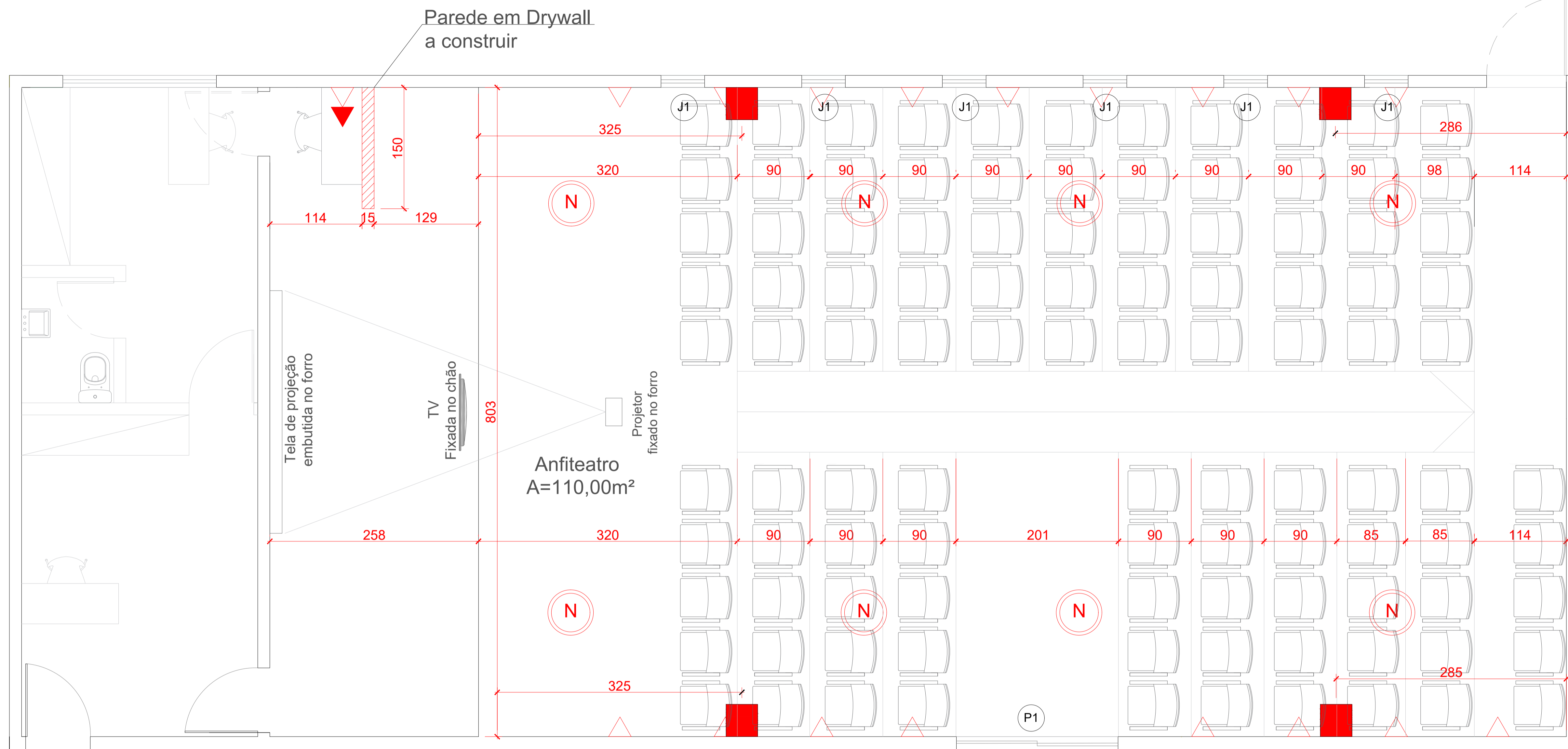
02 PLANTA DE LAYOUT - ANFITEATRO ESC: 1/100
